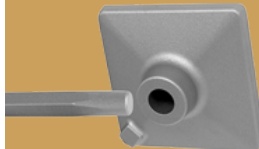
6kt 28x160 Stampplaat 150x150x260mm
